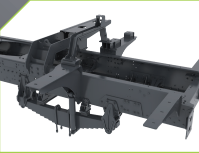
加强型车架 Reinforced frame
